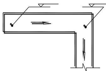
图5 平面图中沟道标高注法
